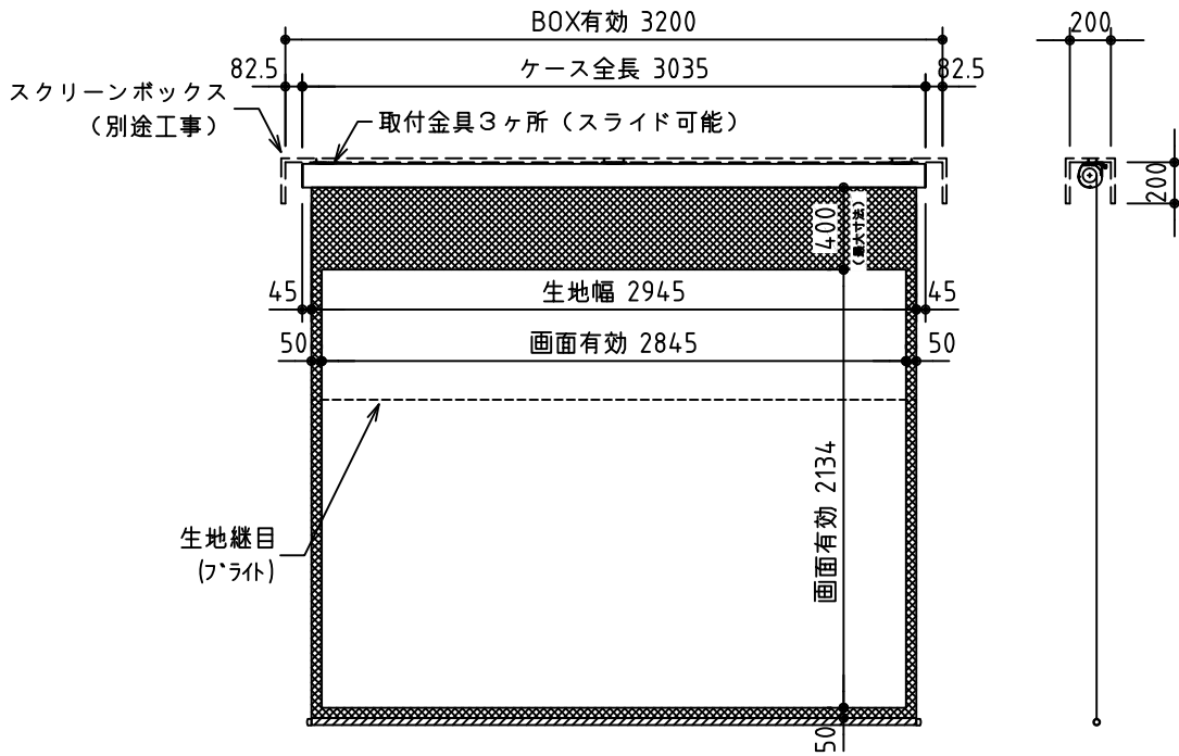
外観図 S=1/40
