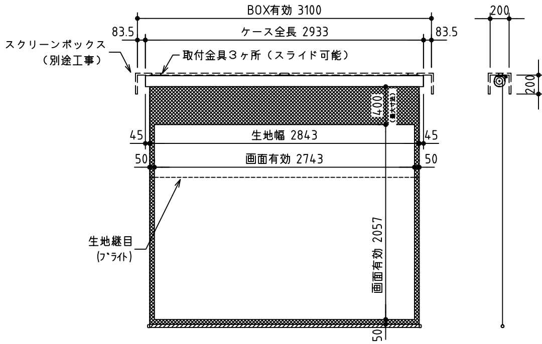
外觀図 S=1/40
