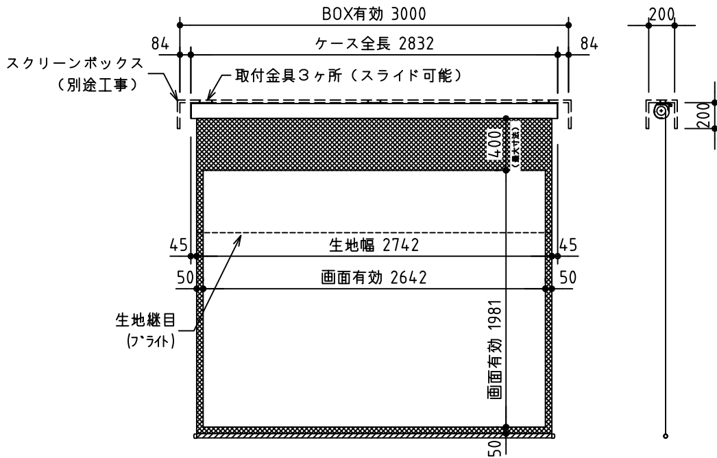
外観図 S=1/40
