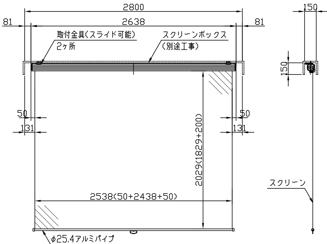
外観図 S=1/30
