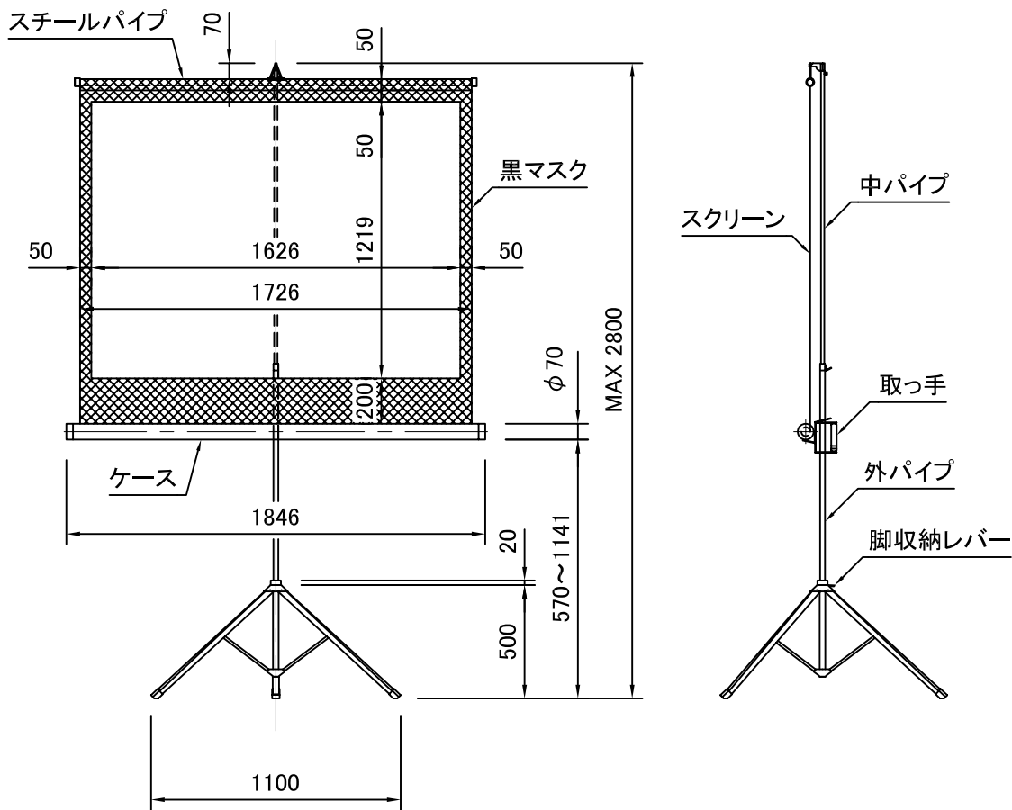
外観図 S=1/30
