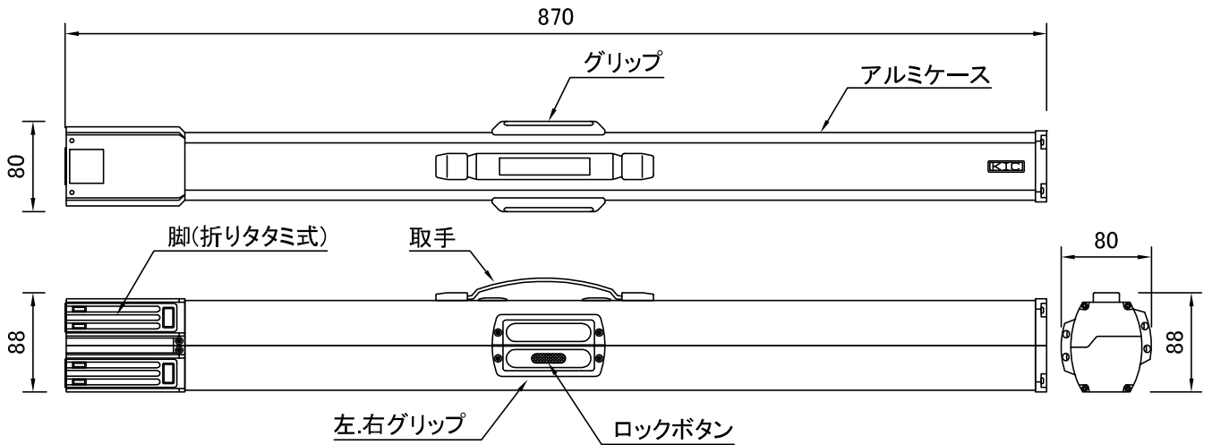
スクリーン収納時ケース外寸 S=1/6
