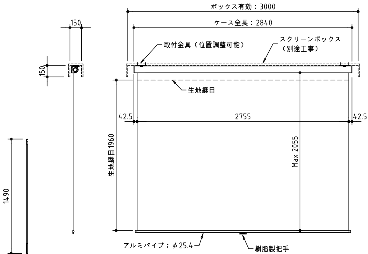
外觀図 S=1/30
