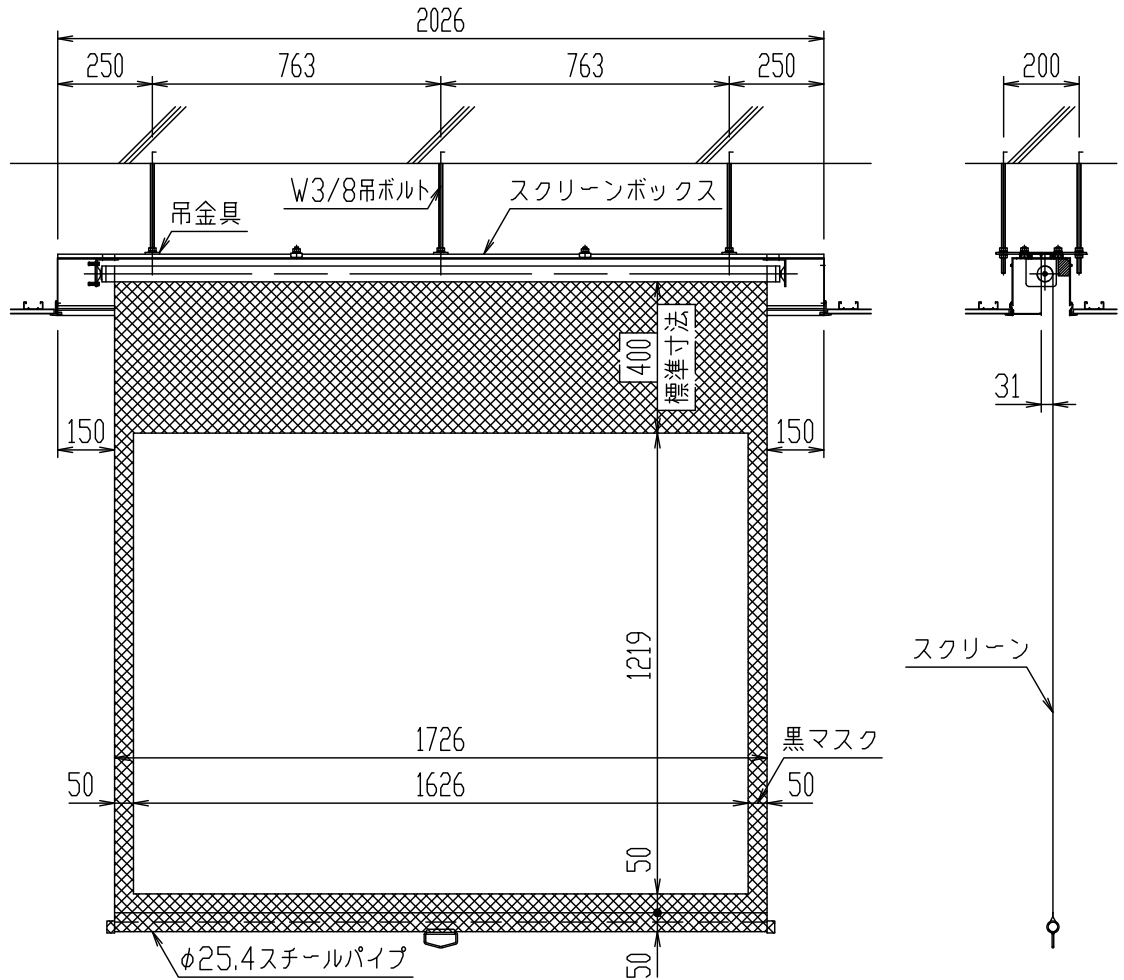
外觀図 S=1/20
