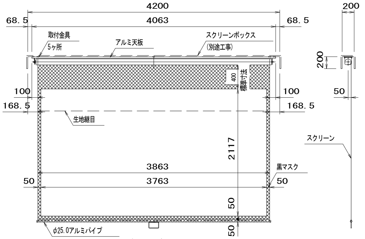
外観図 S=1/40
