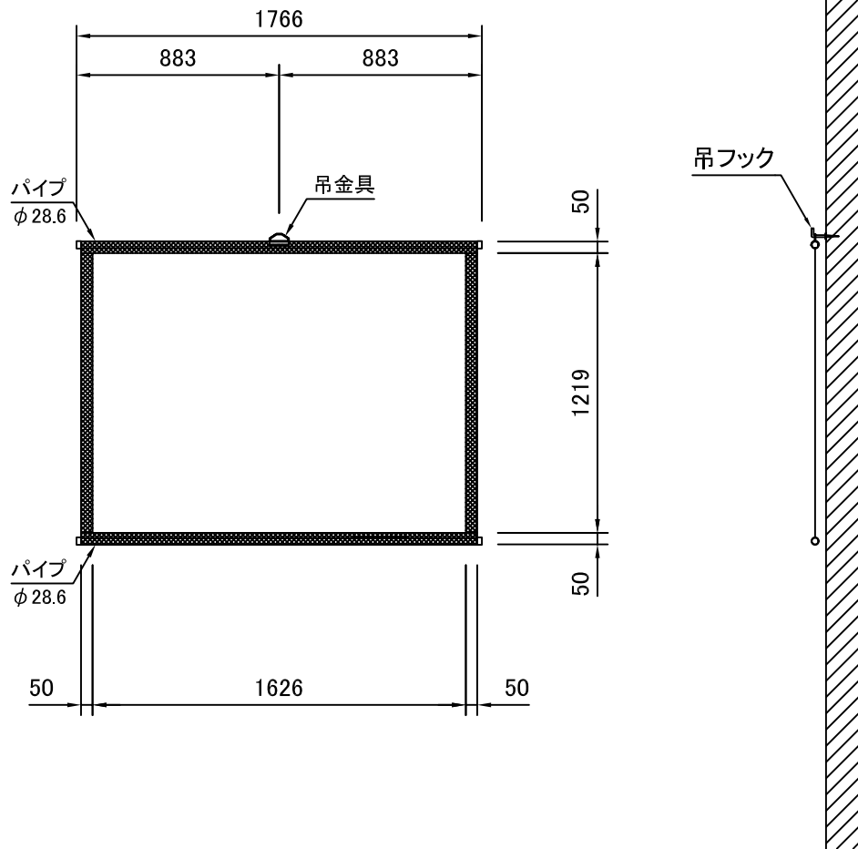
外観図 S=1/30
