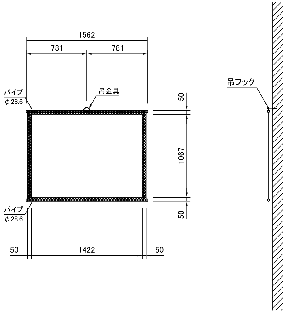
外観図 S=1/30
