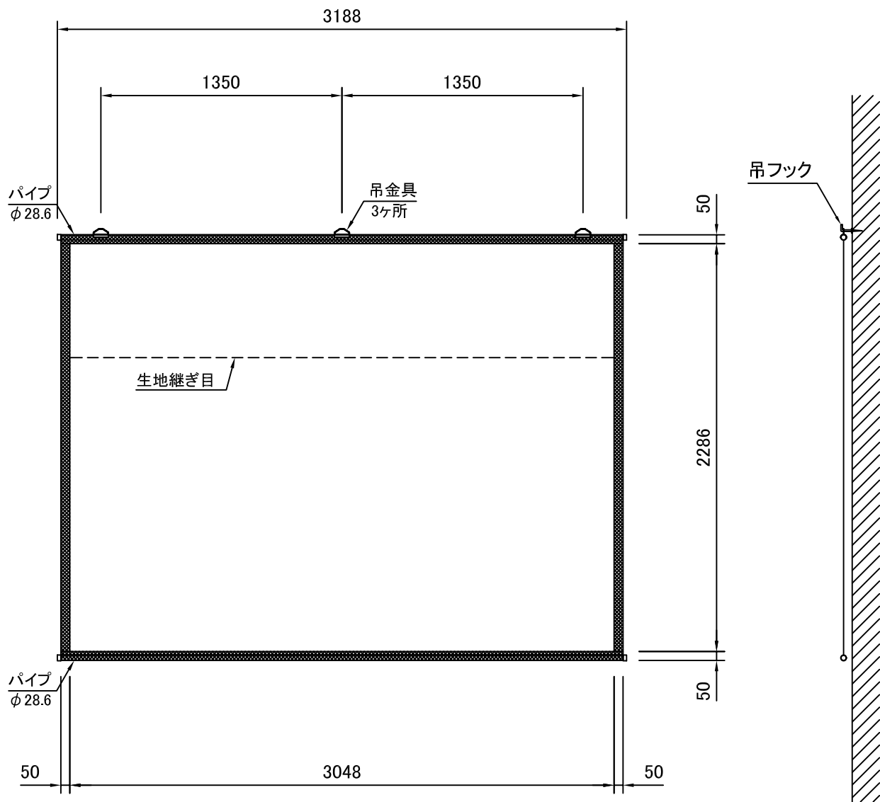
外観図 S=1/30
