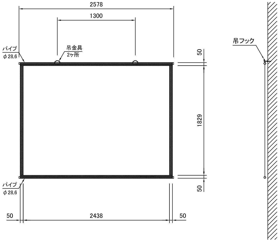
外観図 S=1/30
