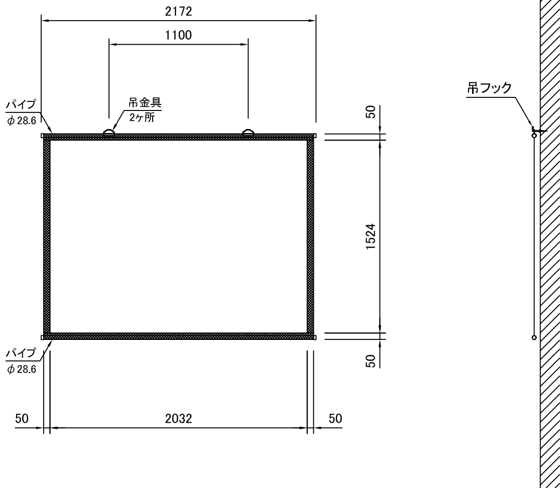
外観図 S=1/30
