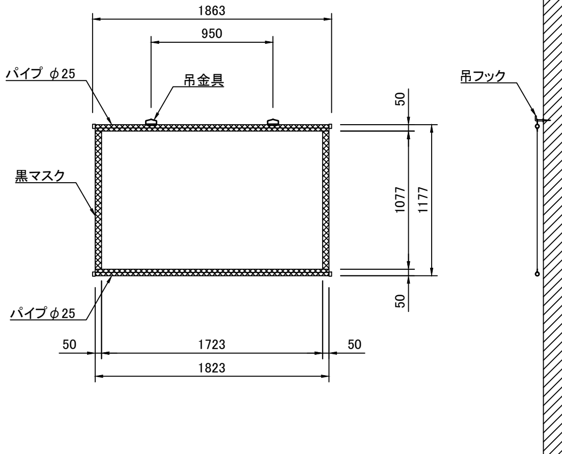
外観図 S=1/30
