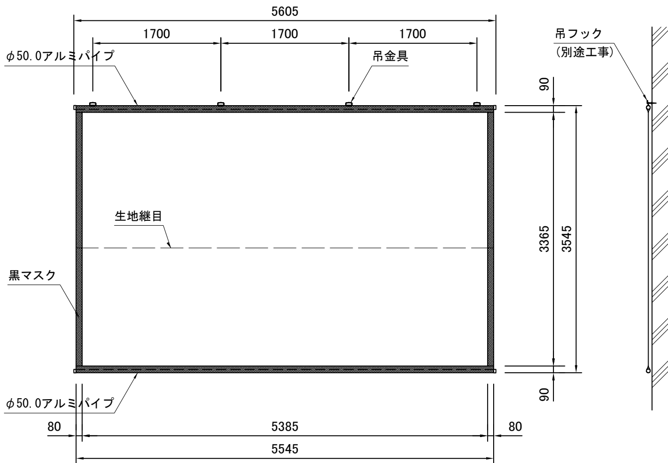
外観図 S=1/50
