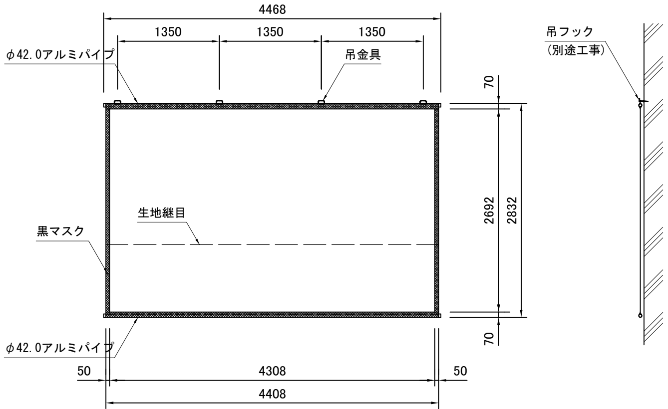
外観図 S=1/50
