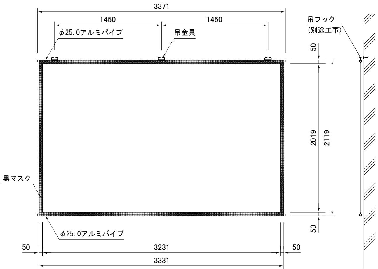
外観図 S=1/30
