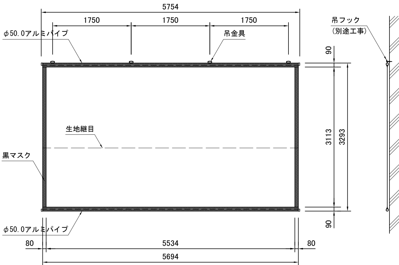
外観図 S=1/50
