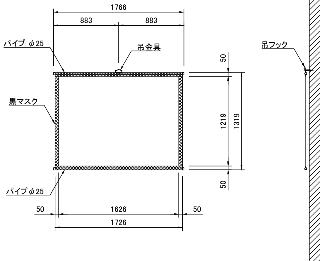
外観図 S=1/30
