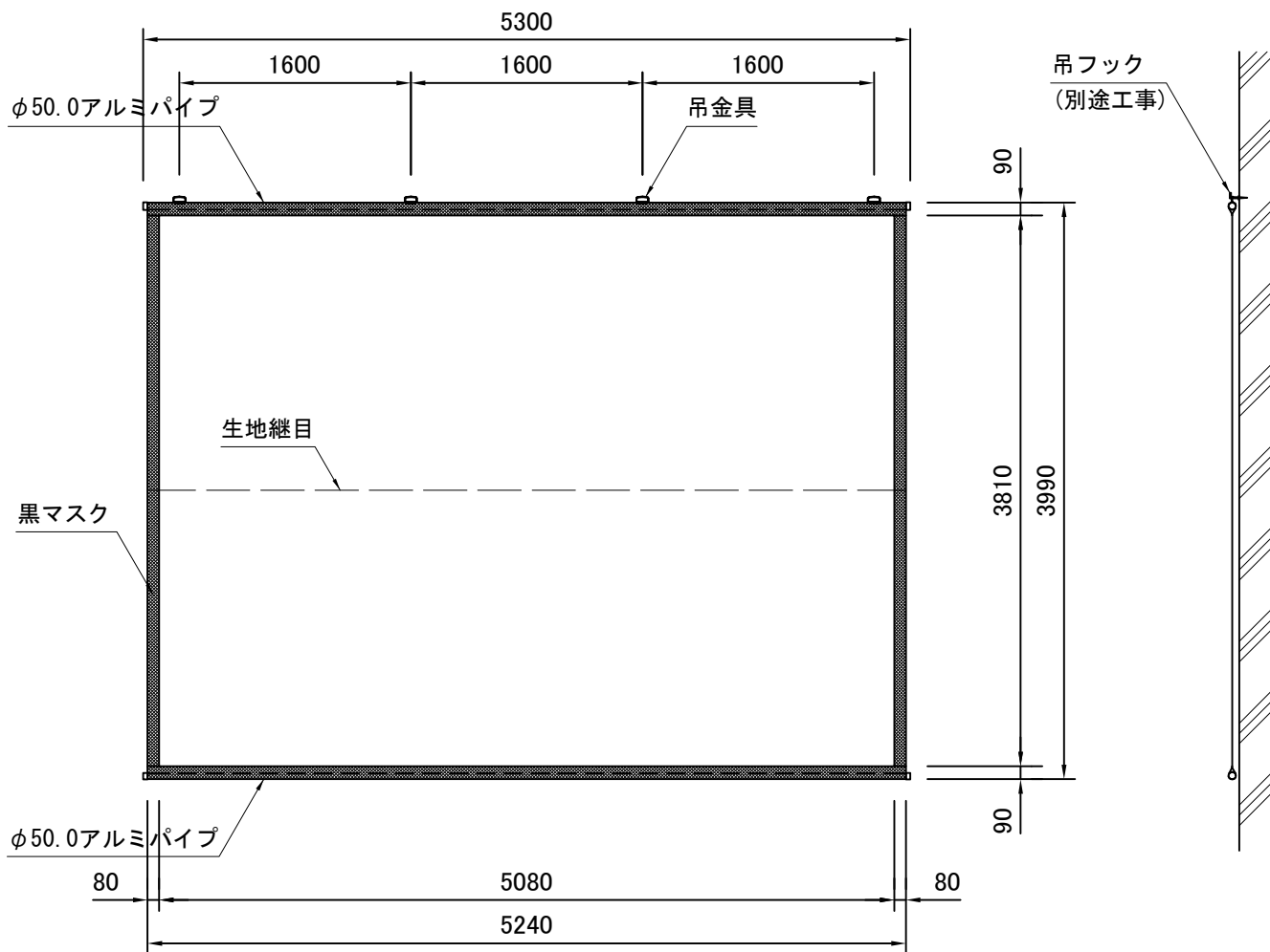
外観図 S=1/50
