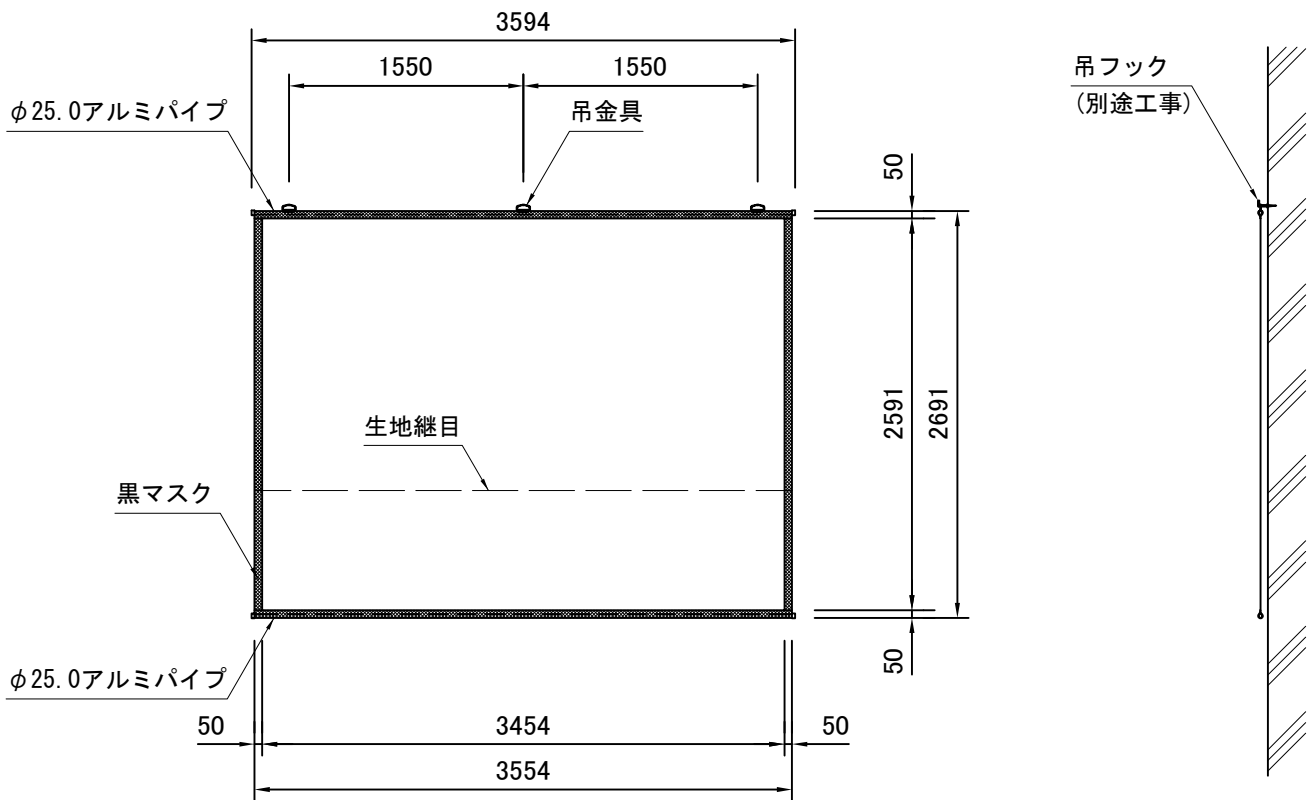
外観図 S=1/50
