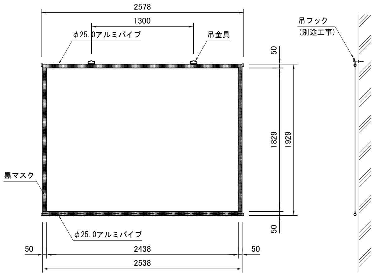
外観図 S=1/30
