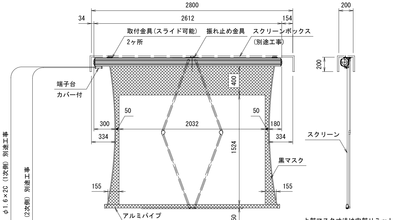
外観図 S=1/30
