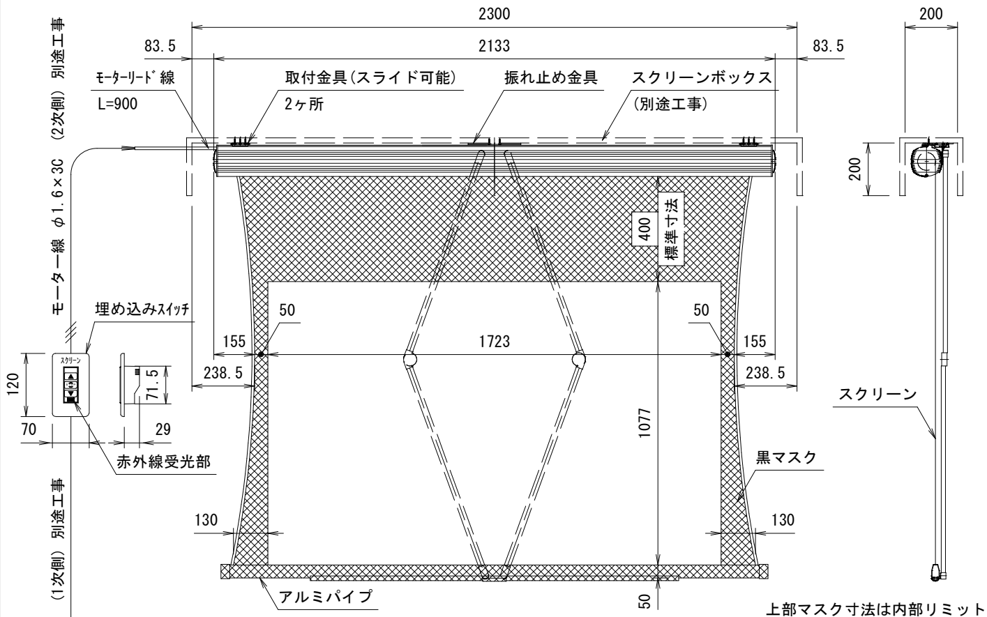
外觀図 S=1/20
