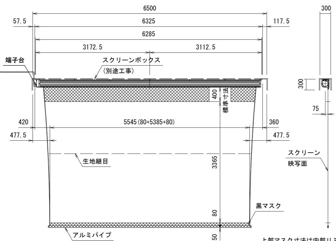
外観図 S=1/60
