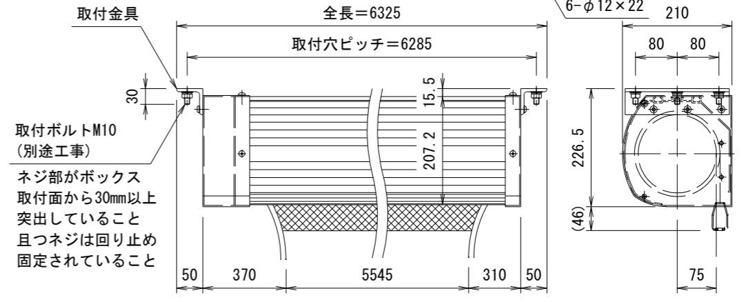
取付部詳細図 S=1/10
