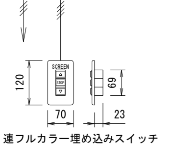
1連フルカラー埋め込みスイッチ
