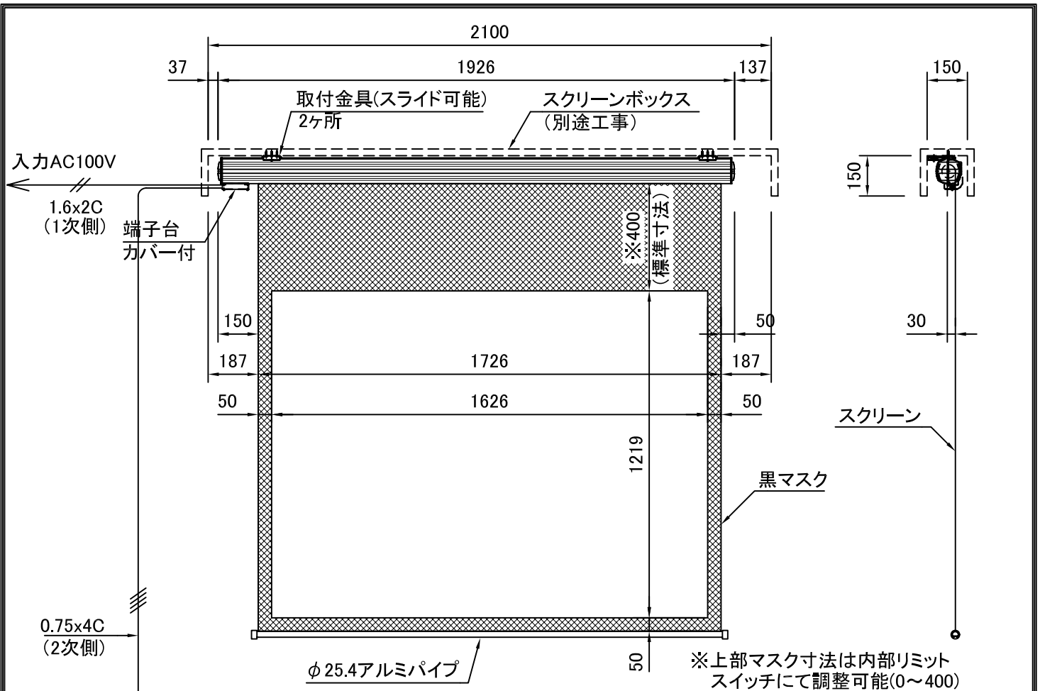
外観図 S=1/20
