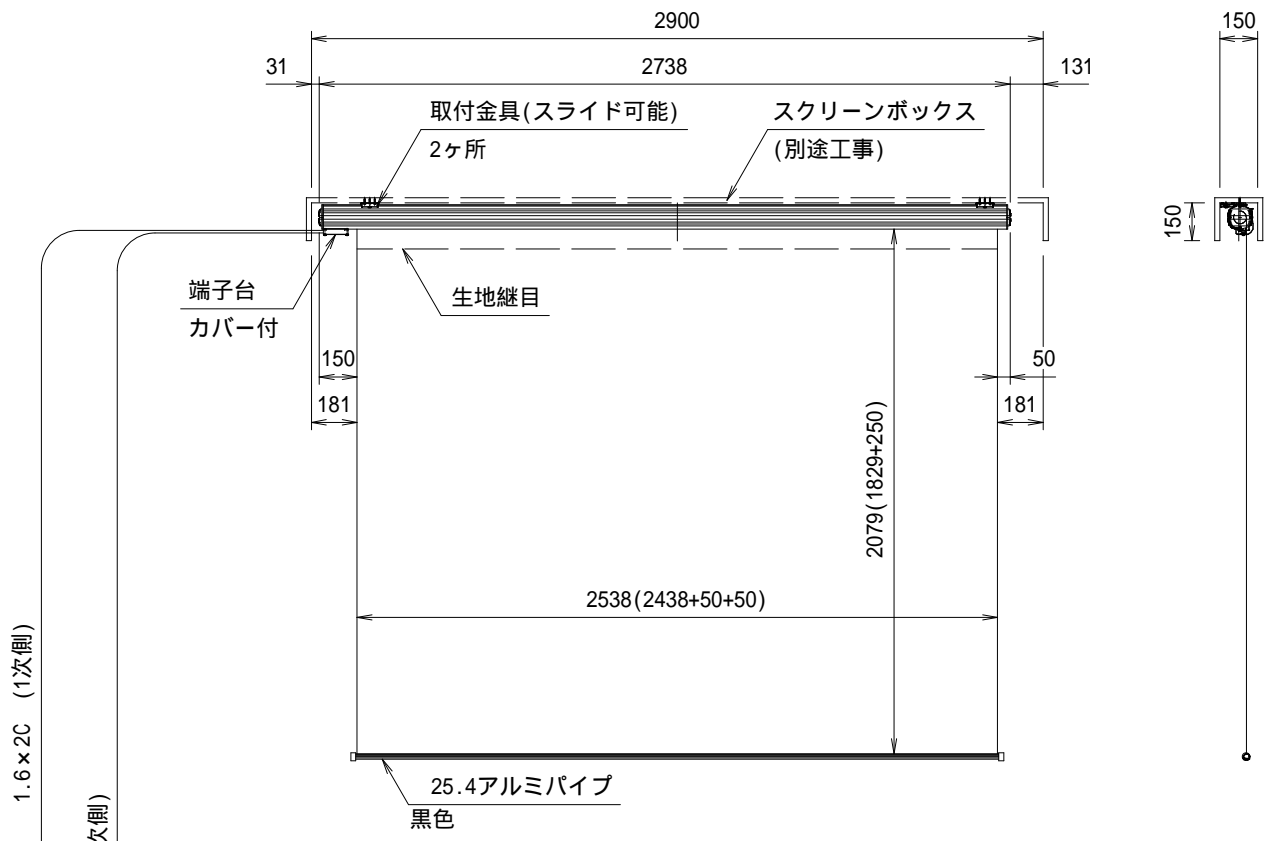
外觀図 S=1/30
