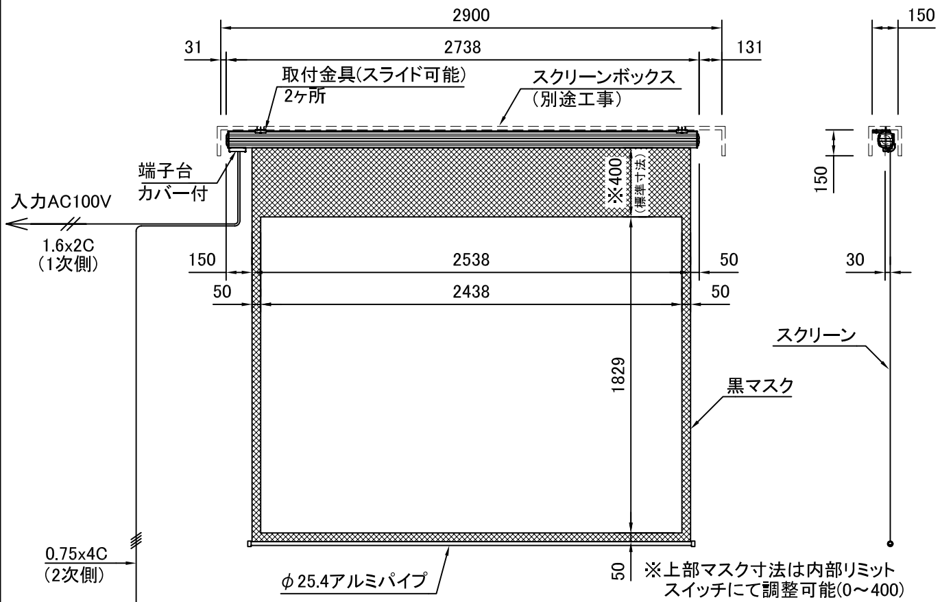
外観図 S=1/30
