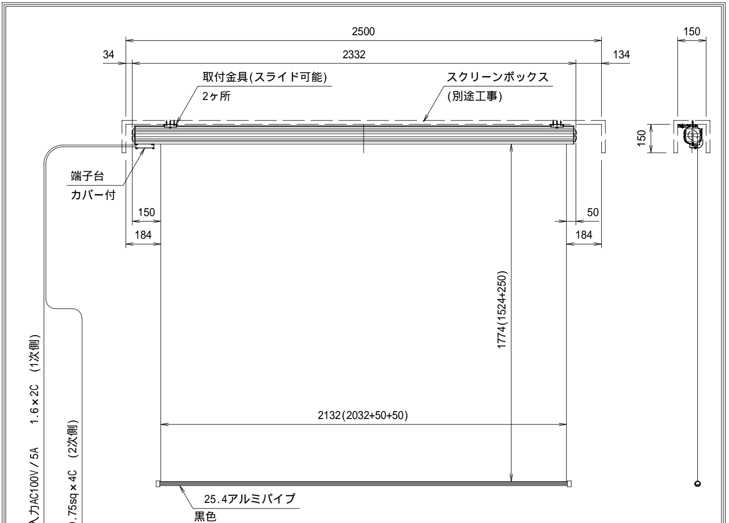
外觀図 S=1/20
