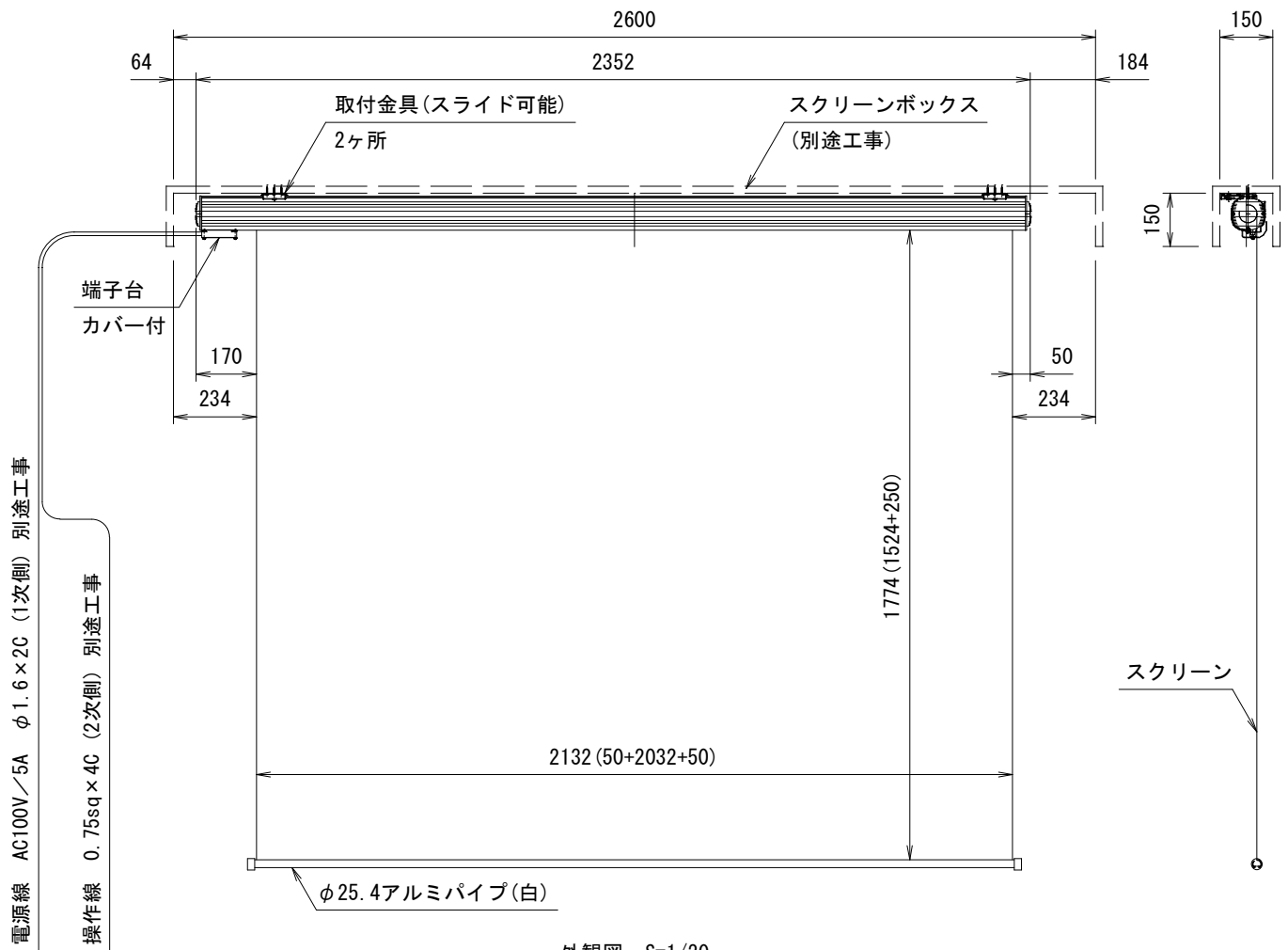
外觀図 S=1/20
