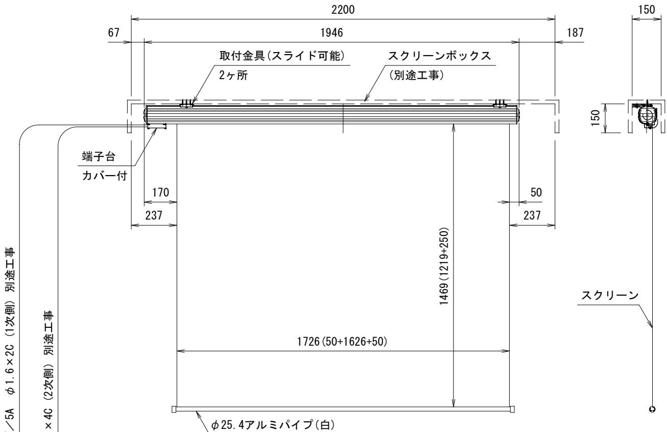
外観図 S=1/20
