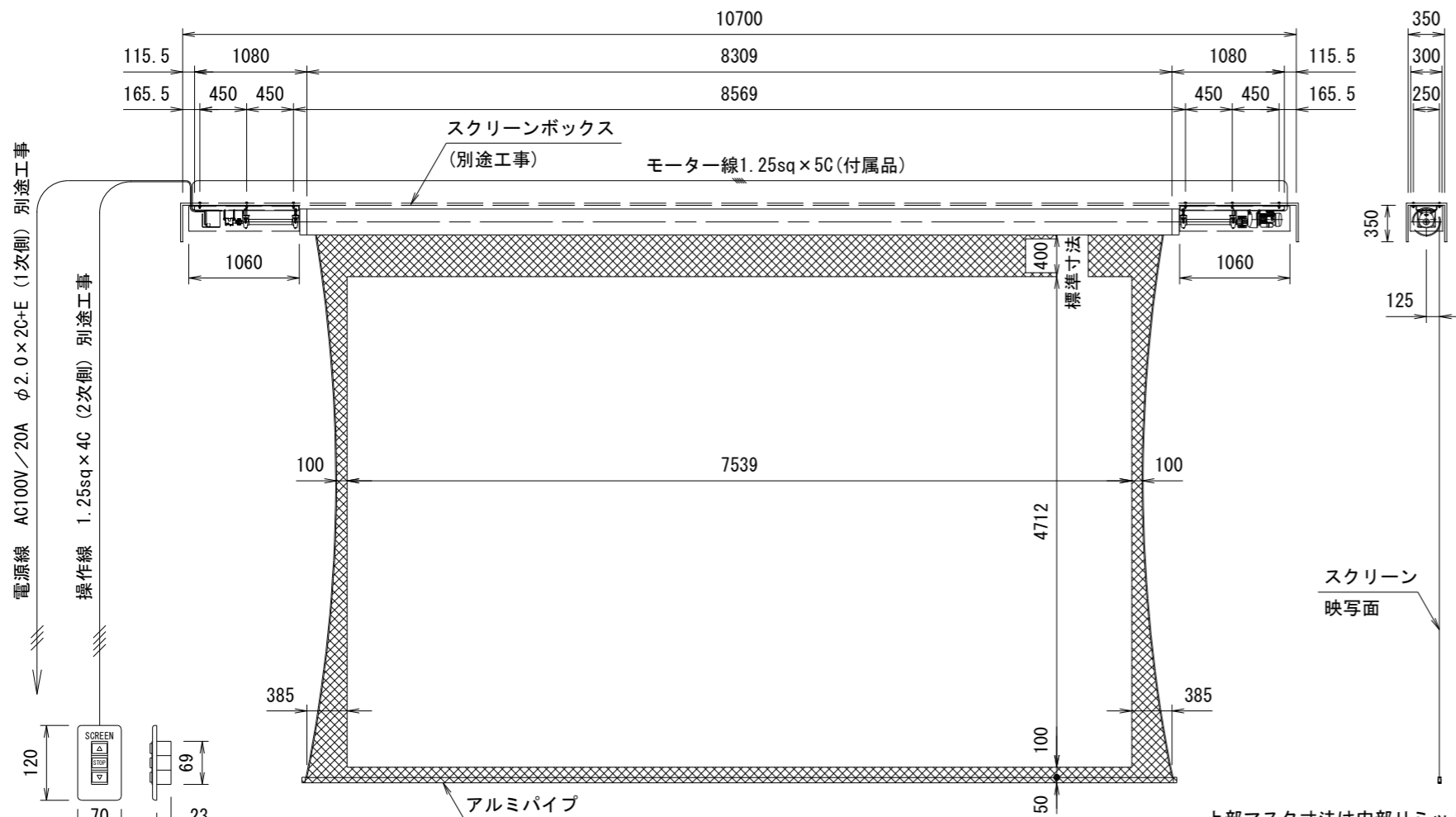
外観図 S=1/60
