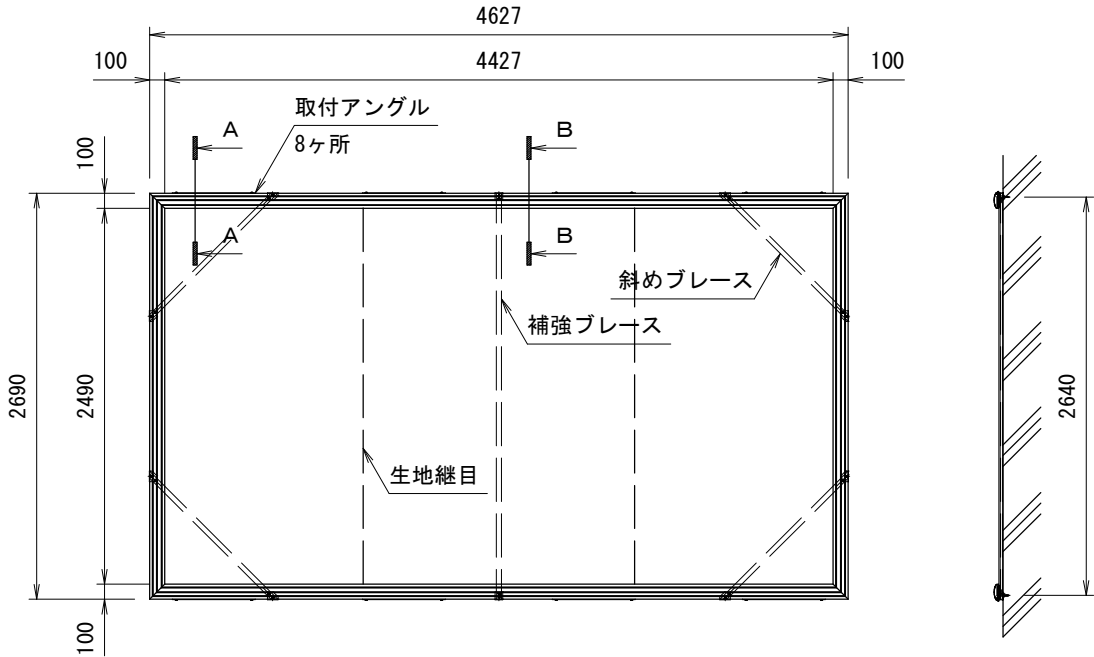
外観図 S=1/50
