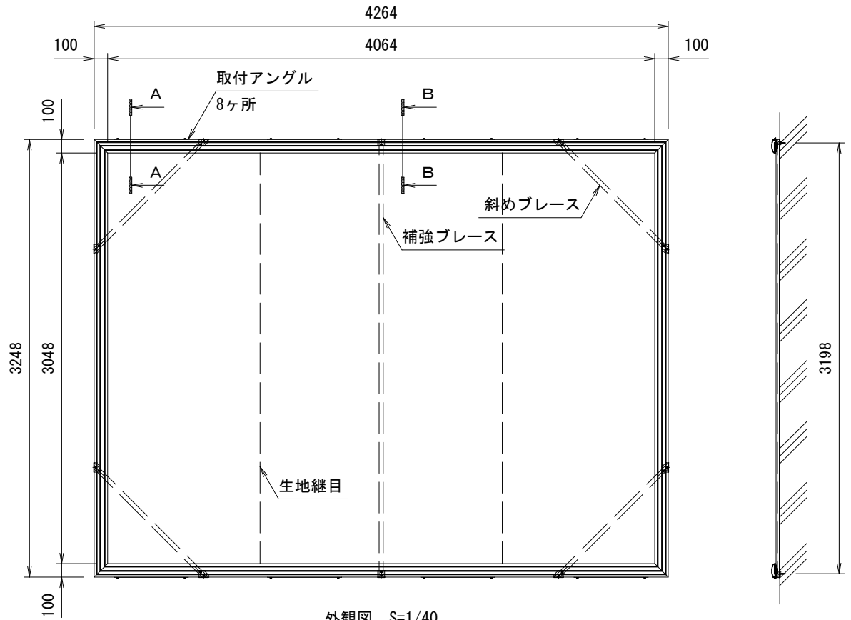
外観図 S=1/40
