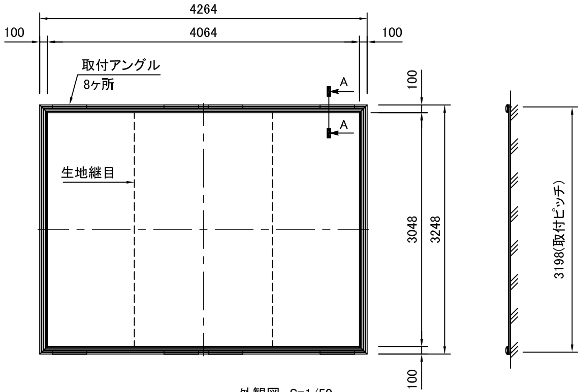
外観図 S=1/50
