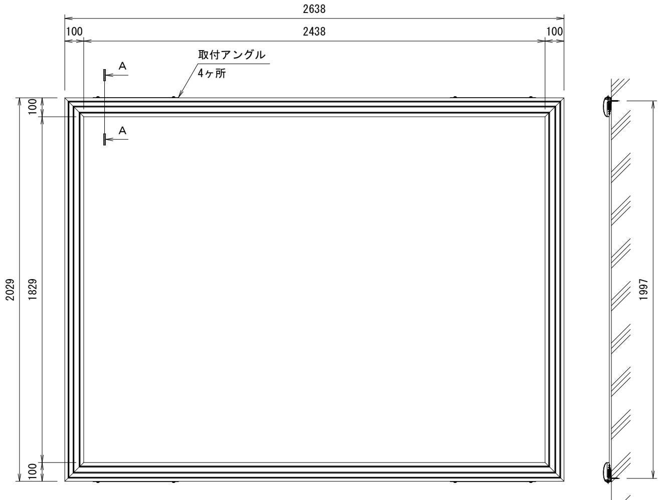
外觀図 S=1/20
