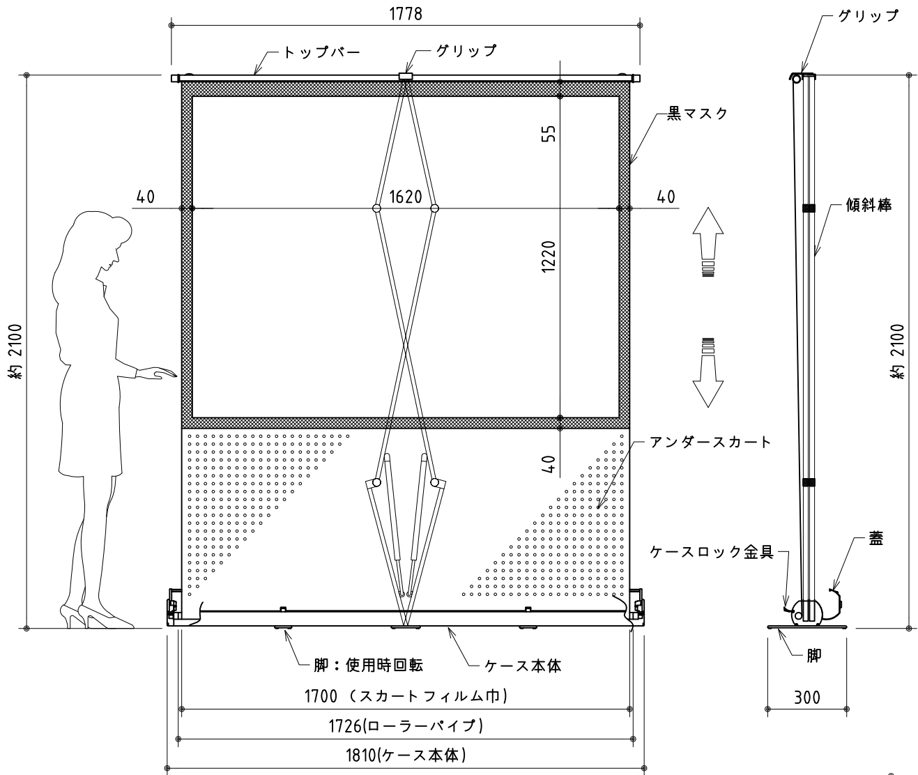
スクリーン設置図 S=1/20
