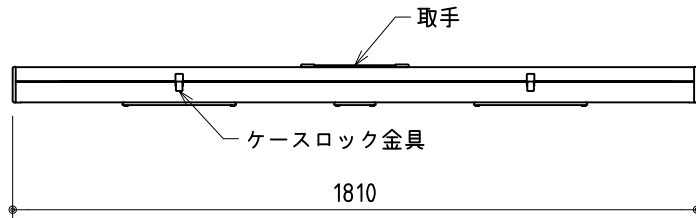
スクリーン収納時ケース外寸 S=1/20
