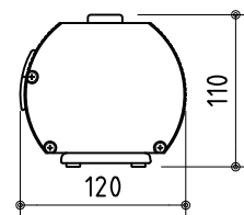
スクリーン収納時ケース外寸 S=1/6
