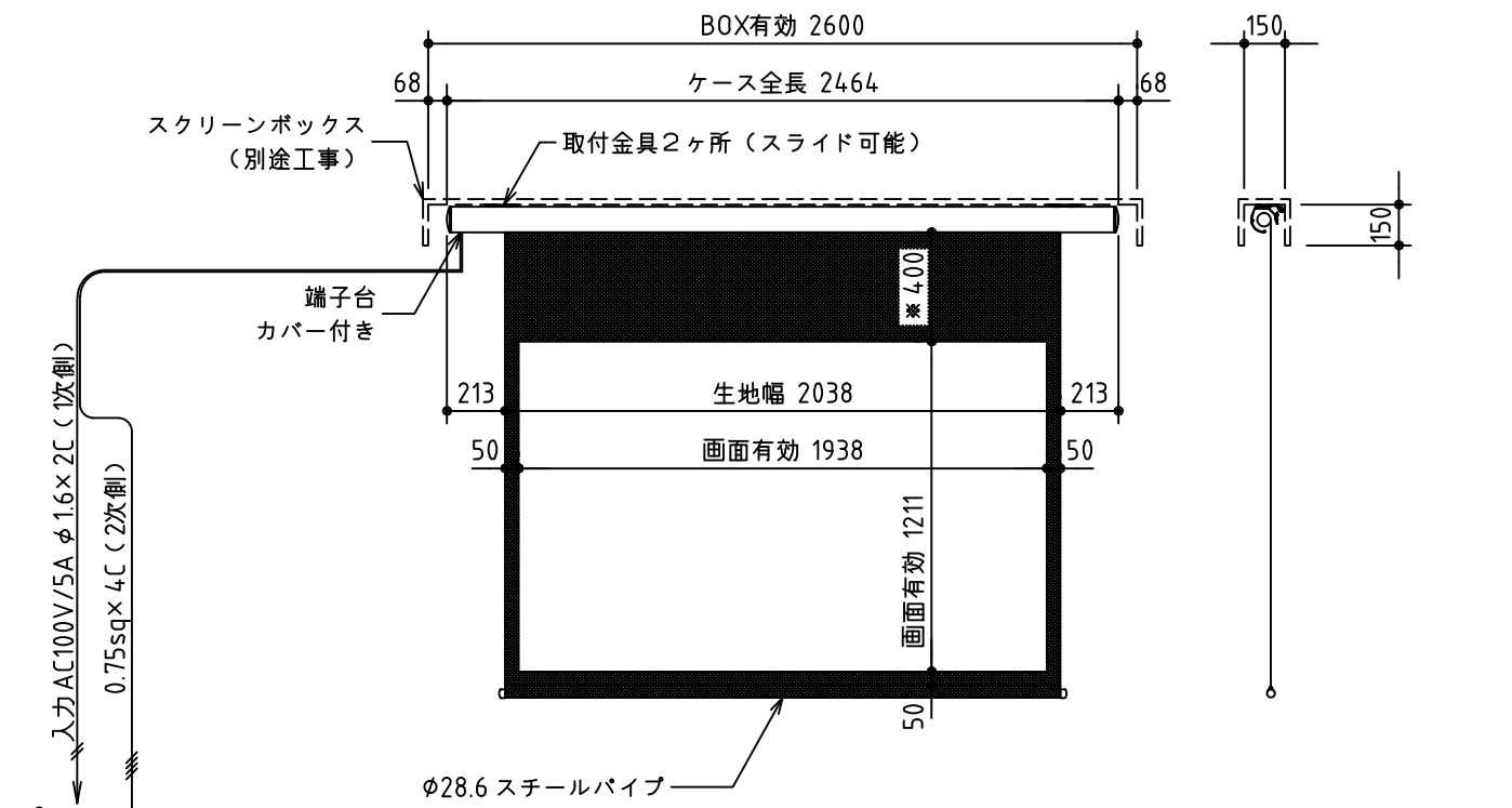
外観図 S=1/30
