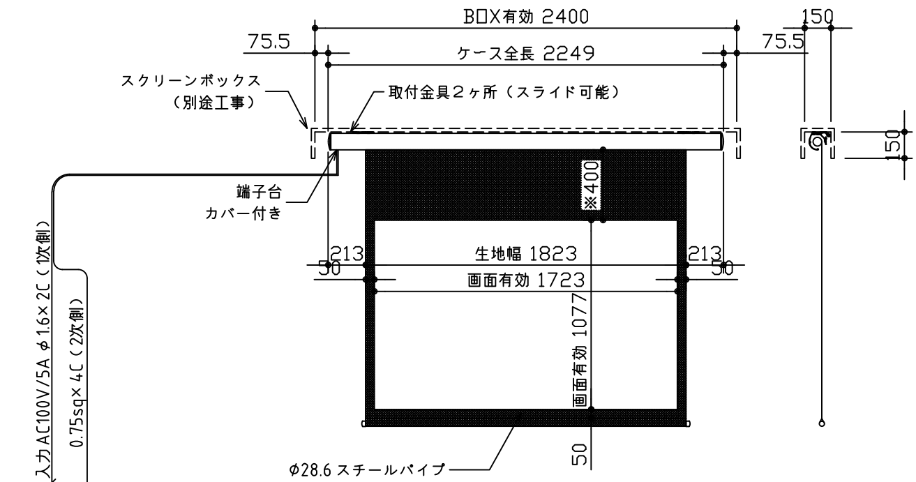
外観図 S=1/30
