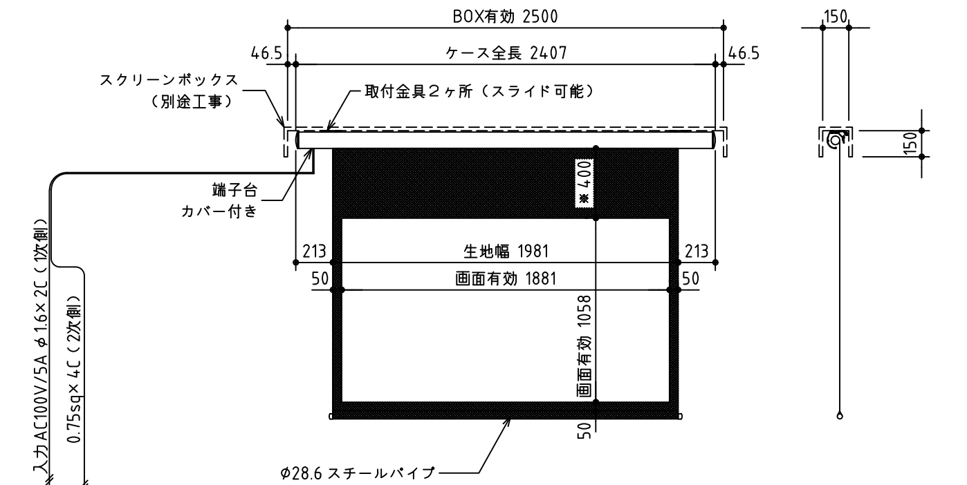
外観図 S=1/30
