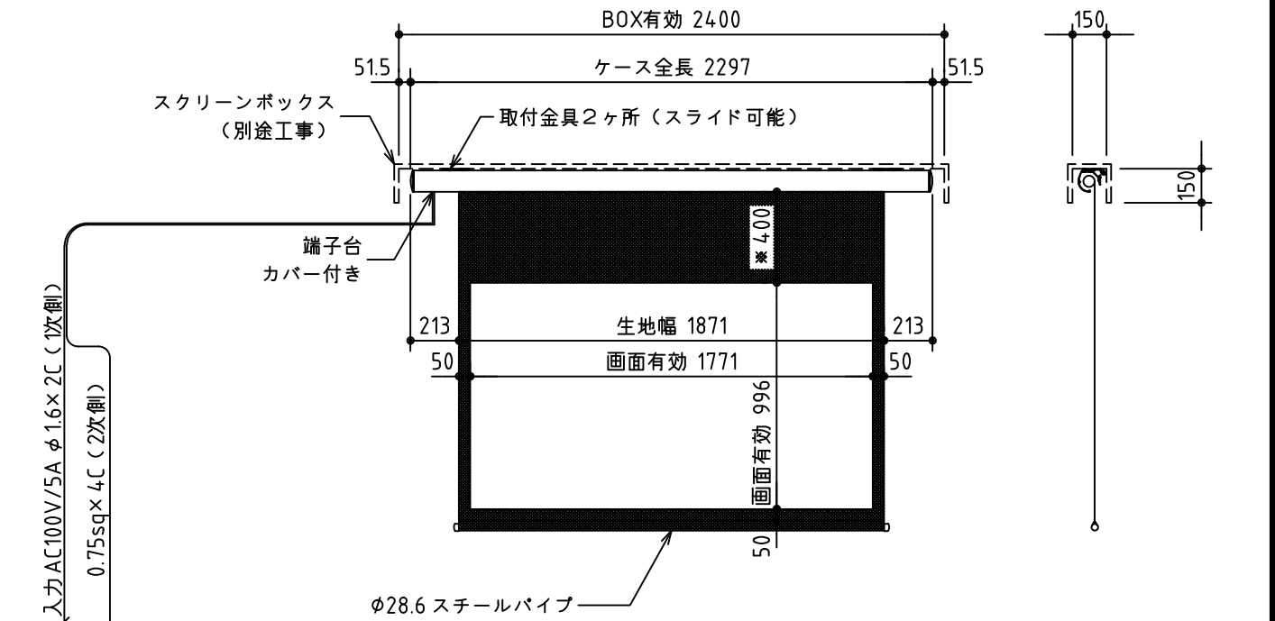
外観図 S=1/30
