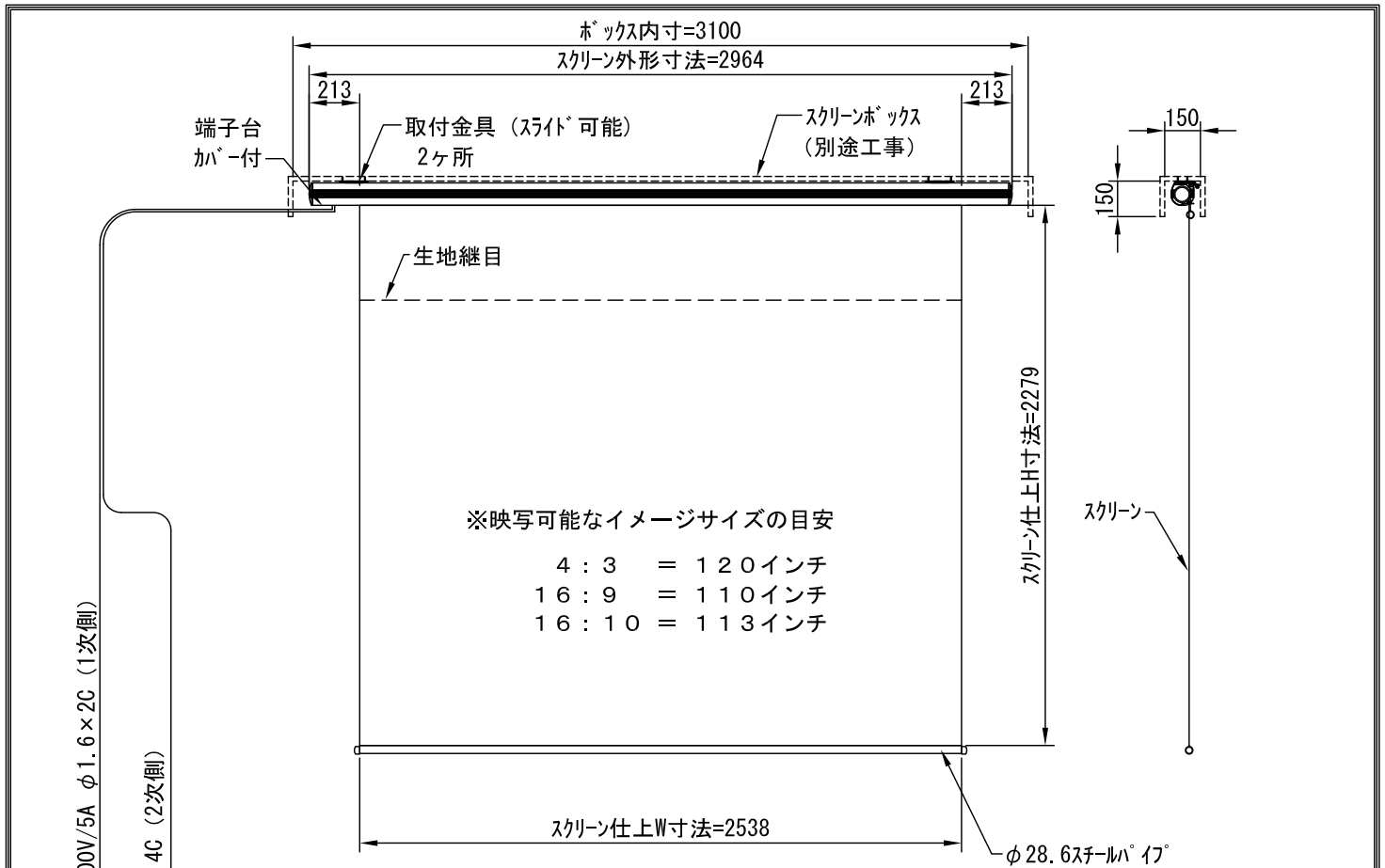
外觀図 1/30
