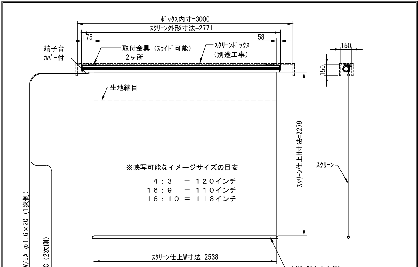
外観図 1/30
