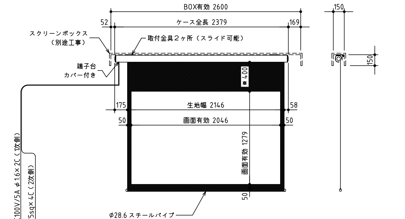
外觀図 S=1/30
