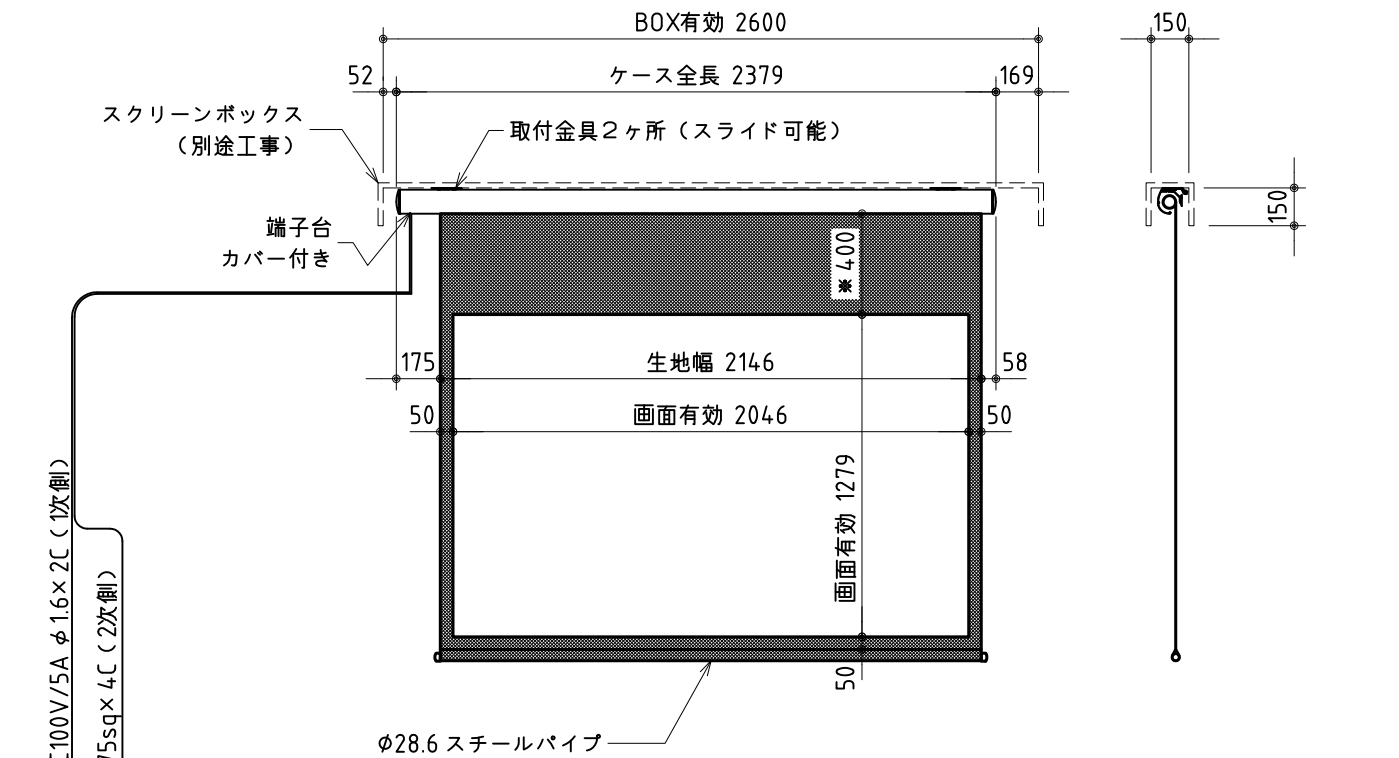
外観図 S=1/30
