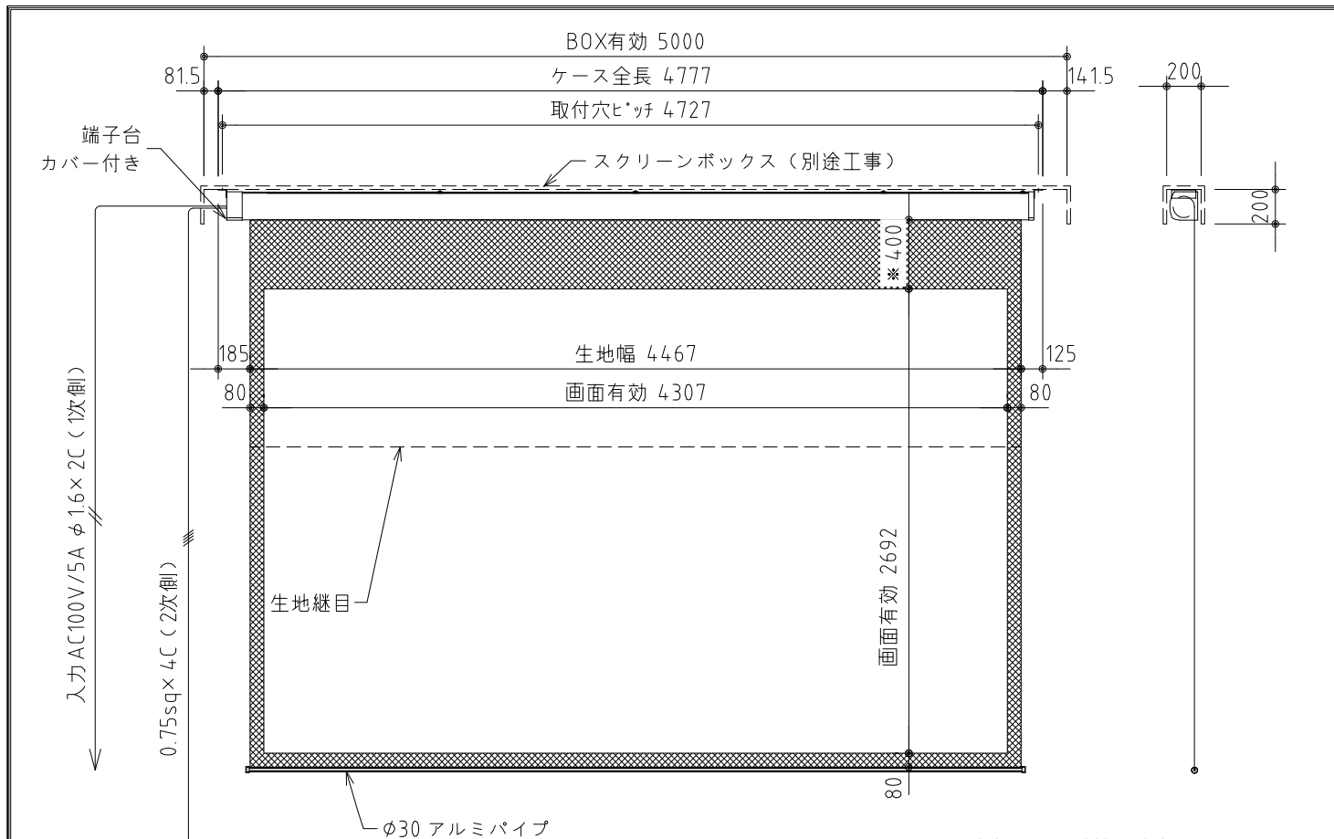
外觀図 S=1/40
