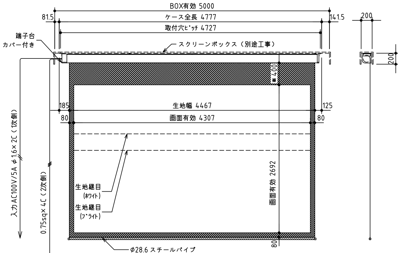
外観図 S=1/40
