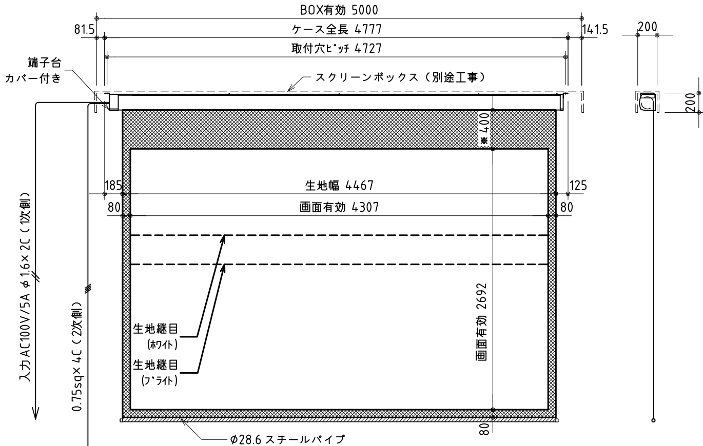
外観図 S=1/40
