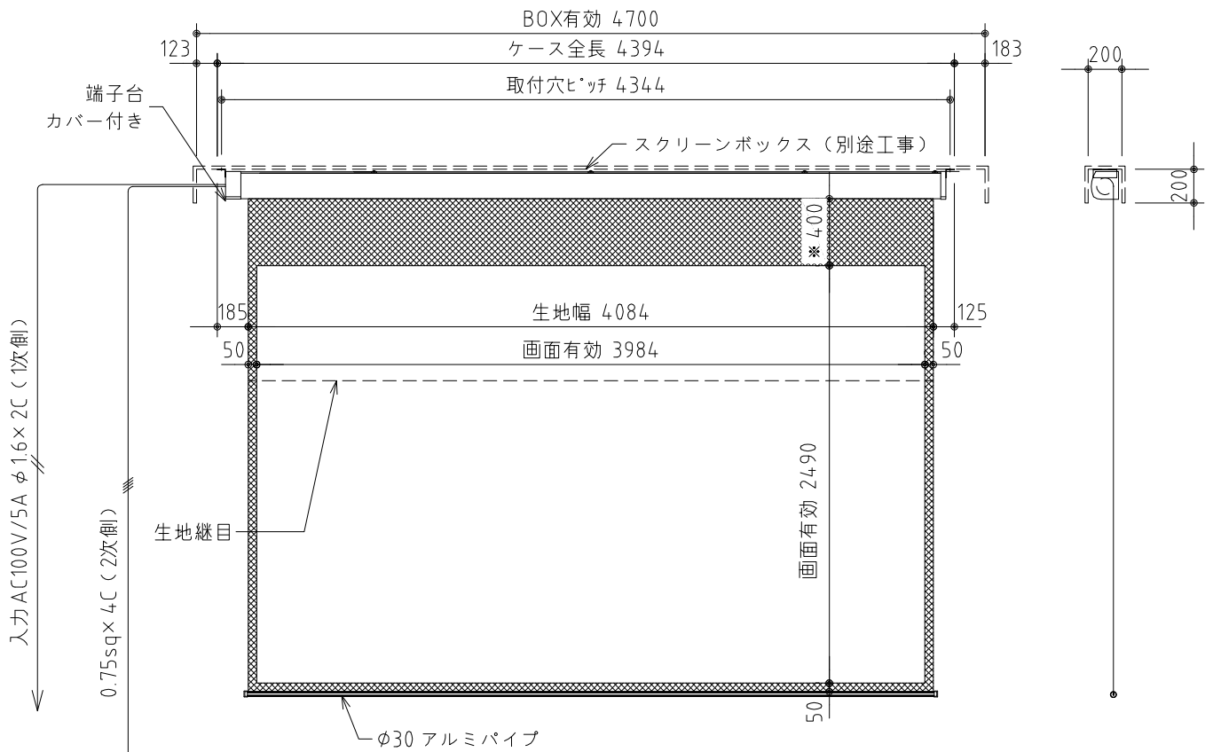
外觀図 S=1/40
