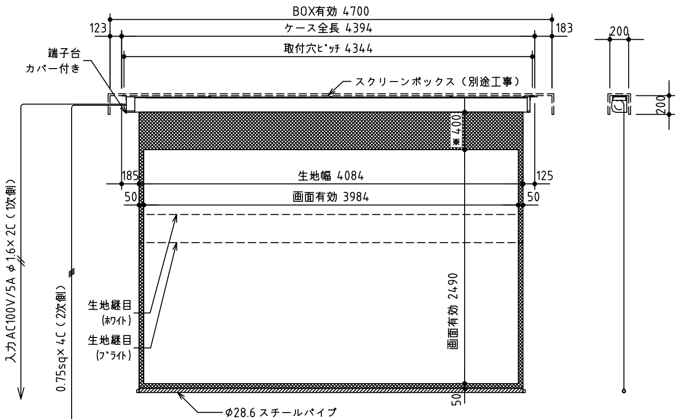
外観図 S=1/40
